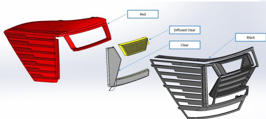
Bezel
